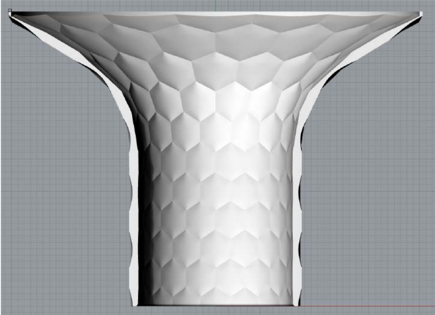
Hex table
